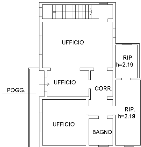
Piano Primo H=2,74
